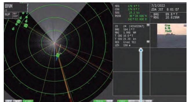
周囲情報統合システム 画面例
